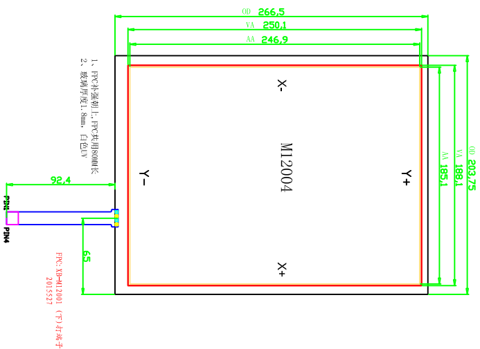
正视图
